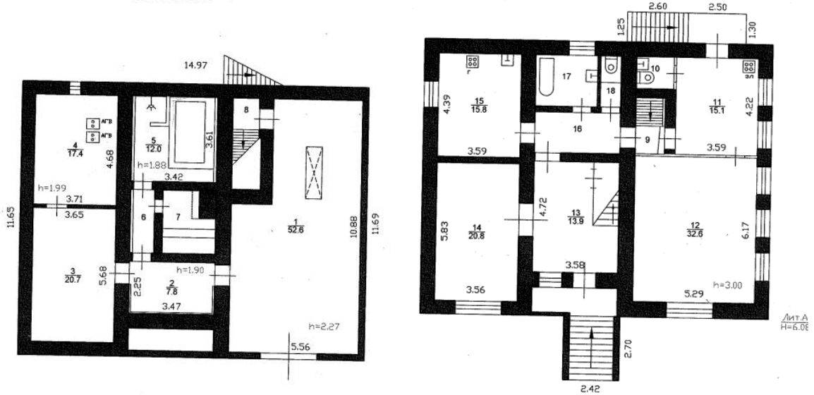
Цокольный этаж
