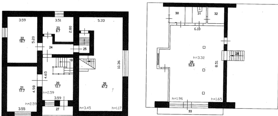
2 этаж
